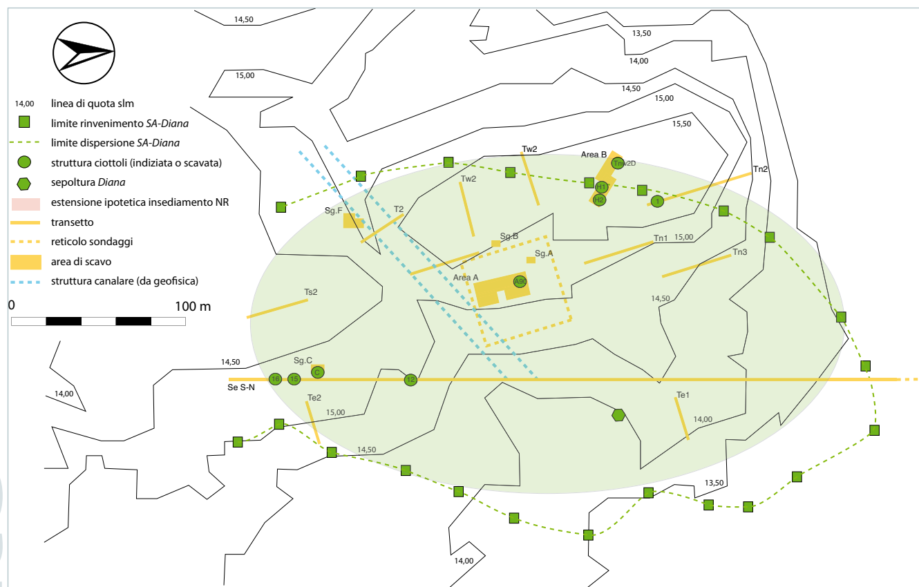
Figura 1 - Favella. Planimetria schematica del villaggio nel Neolitico recente.
